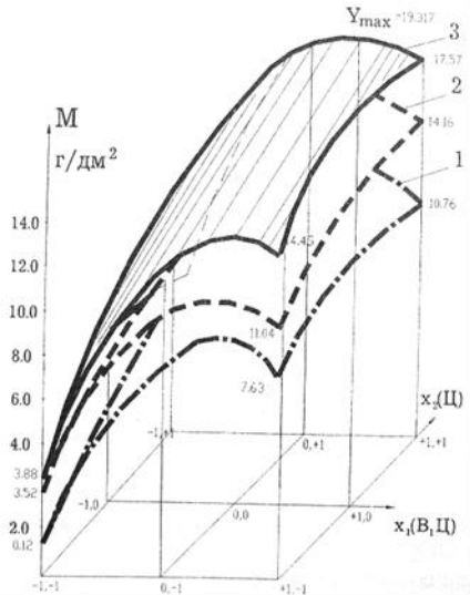
Рисунок 2 – Массопоглощение в зоне контакта: 1 – при x_3 = +1 ; 2 – при x_3 = 0 ; 3 – при x_3 = -1 .
