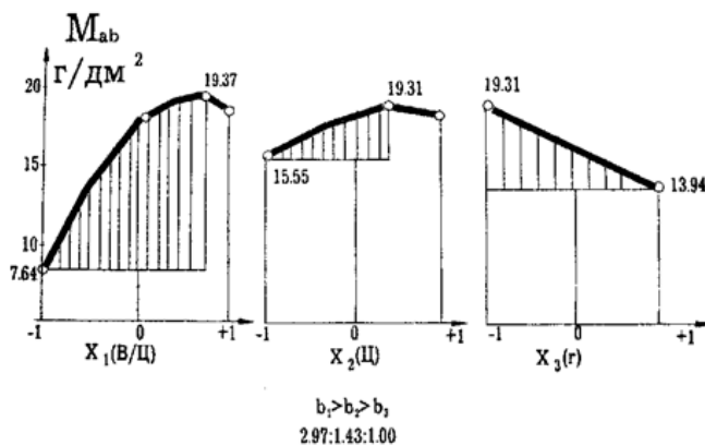
Рисунок 4 – Однофакторные зависимости M_{ab} и распределение факторов по рангам влияния.
