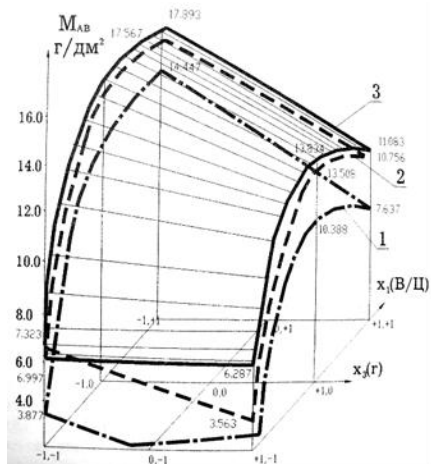
Рисунок 3 – Зависимость массопоглощения от \gamma и от В/Ц: 1 – при C = 300 \text{ кг/м}^3 ; 2 – при C = 400 \text{ кг/м}^3 ; 3 – при C = 500 \text{ кг/м}^3 .
