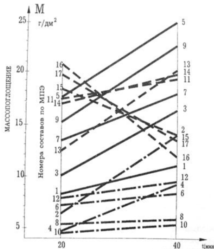
Рисунок 1 – Изменение величины массопоглощения во времени:
