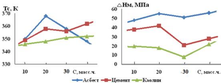
Рис.2. Влияния содержания асбеста, цемента и каолина на температуру стеклования ( T_g ) и прочности ( \Delta H ) ГКПМ на основе ЭД-16.
