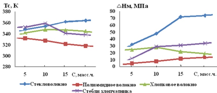
Рис.4. Влияния содержания асбеста, цемента и каолина на температуру стеклования ( T_c ) и прочности ( \Delta H ) ГКПМ на основе ЭД-16.
