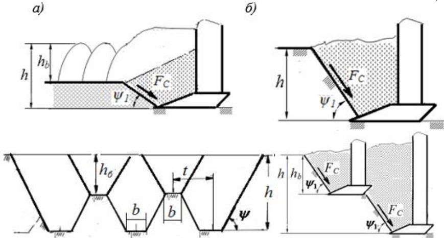
Рисунок -3. Схема последовательности разрушения уплотненной почвы подпахотного горизонта и силы скалывания
