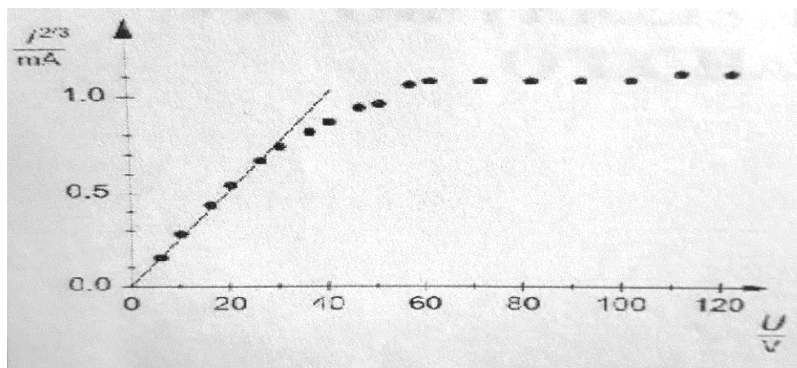
5-rasm. Hajmiy zaryadlarning chegaralash sohasi I^2/3A anod kuchlanishi UA ning funksiyasi sifatida. Lengyur-Chayld tenglamasiga asosan natija to'g'ri chiziqdan iborat bo'ladi.
