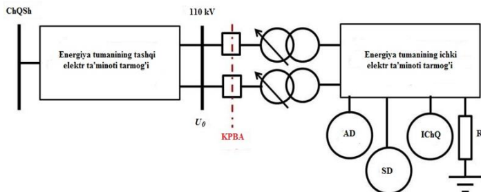
1-rasm. Energiya tumanining tashqi aloqali soddalashtirilgan hisobli sxemasi
