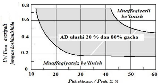
4-rasm. Yuklama tarkibining o'zgarishidan kelib chiqib muvaffaqiyatli bo'linish hududi chegarasi holatining grafik bog'liqligi ko'rinishi
