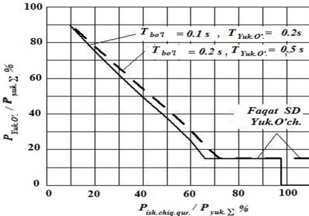
2-rasm. Ishlab chiqaruvchi qurilmaning har xil umumiy quvvatlarida zarur bo'lgan yuklamani o'chirish hajmlarining jadvali.
