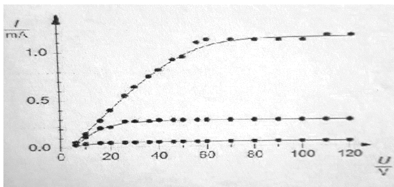
4-rasm. Qizdirish kuchlanishining uch har xil qiymati U_1 , U_2 , va U_3 lar uchun anod toki IA ning anod kuchlanishi UA dan bog'liqligi.
