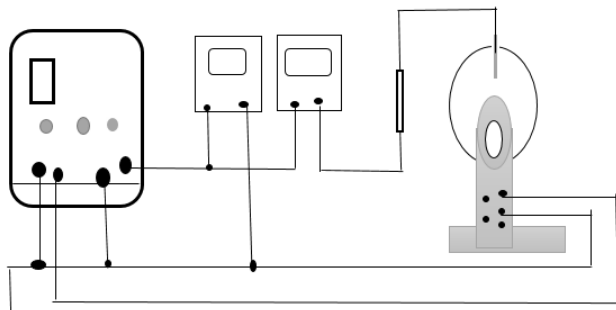
3-rasm. Diodning xarakteristikasini o'lchash uchun eksperimental qurilma [5].
