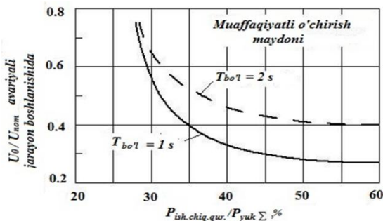
3-rasm. KPBA javob tezligining qo'shimcha yuklamani o'chirishsiz muvaffaqiyatga erishish ta'sirining grafigi
