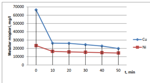
1-rasm. NH_4CNS ni qo'llab mis va nikelni eritmadan cho'ktirish jarayonini vaqtga bog'liqlik grafigi.
