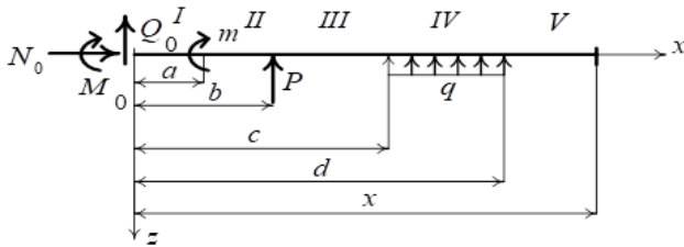
Сурет 1. Арқалықтың иілуі
